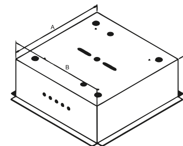
PLAFON PRISMA G PE 1111 De Embutir Alt.: 21 cm Base: 26 cm Comp.: 8 cm Vidro: 34 x 44 cm Soquete E 27
