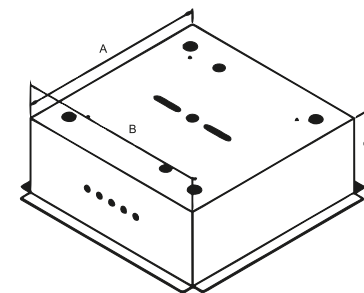
PLAFON PRISMA P PE 1110 De Embutir Alt.: 20 cm Base: 20 cm Comp.: 8 cm Vidro: 30 x 30 cm Soquete E 27
